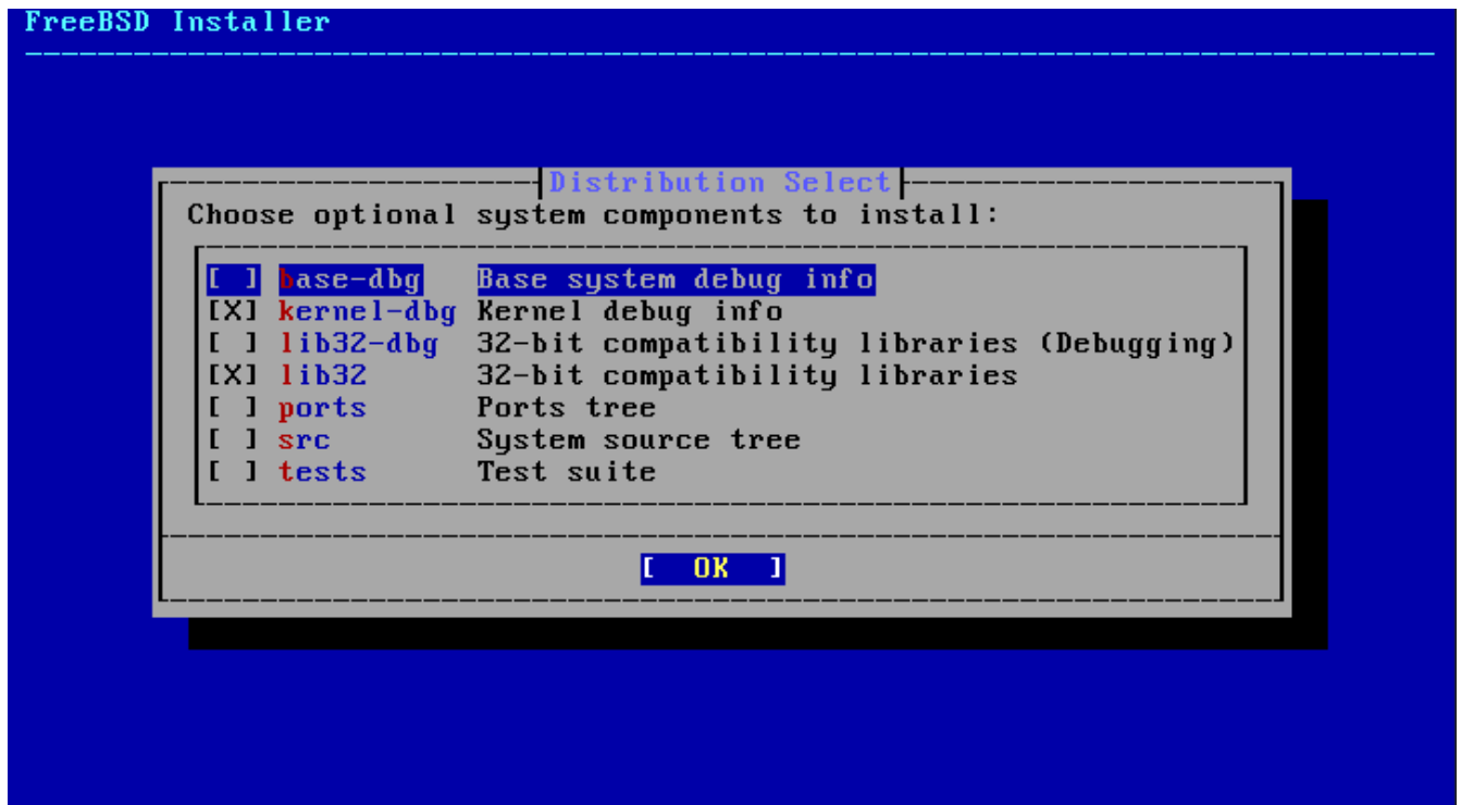
图 64. 选择要安装的组件
