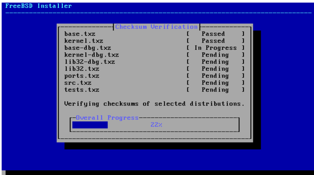
图 76. 验证组件对应的文件
