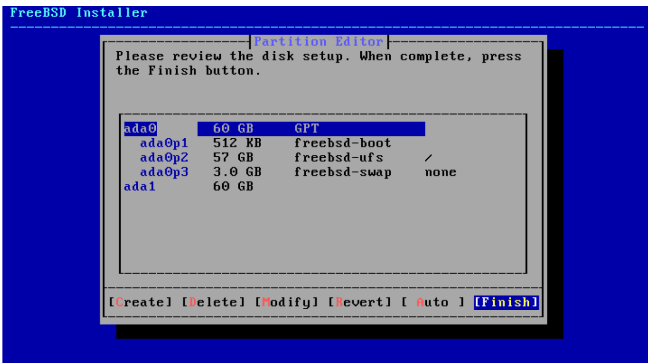
图 70. 检查已创建分区
