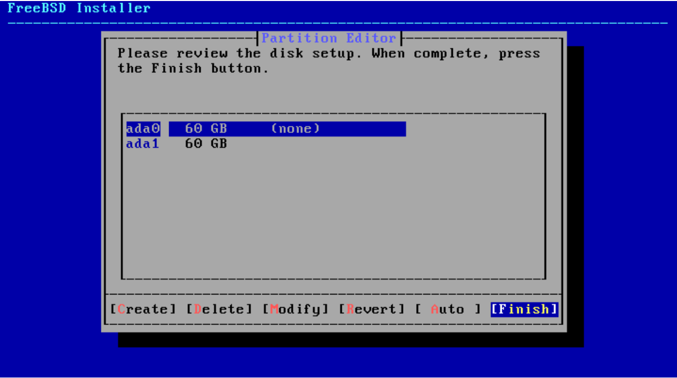
图 71. 手动创建分区
