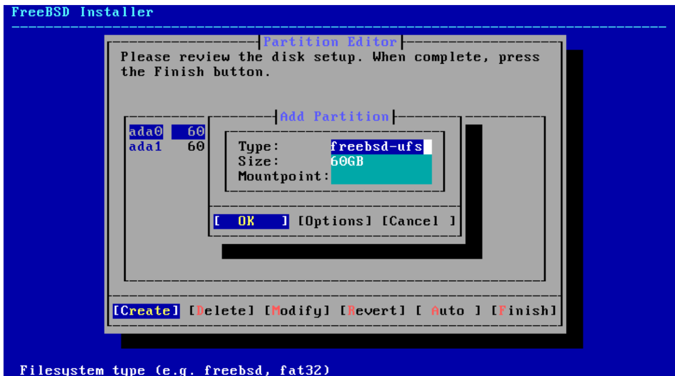
图 73. 手动创建分区
