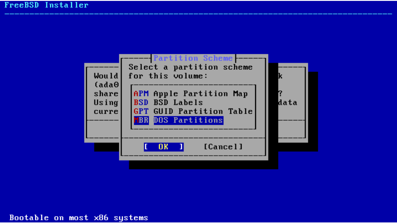
图 72. 手动创建分区
